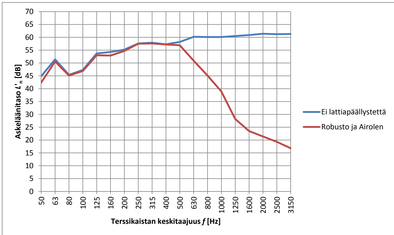
Kuva 1. Ilman lattiapäällystettä sekä laminaatilla Robusto ja askeläänieristeellä Airolen fc combi mitatut askeläänitason spektrit.
